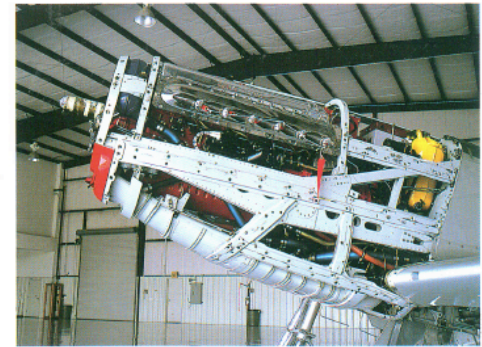
De twaalfcilinder Merlin van een van de zusterschepen van Crazy Horse.
